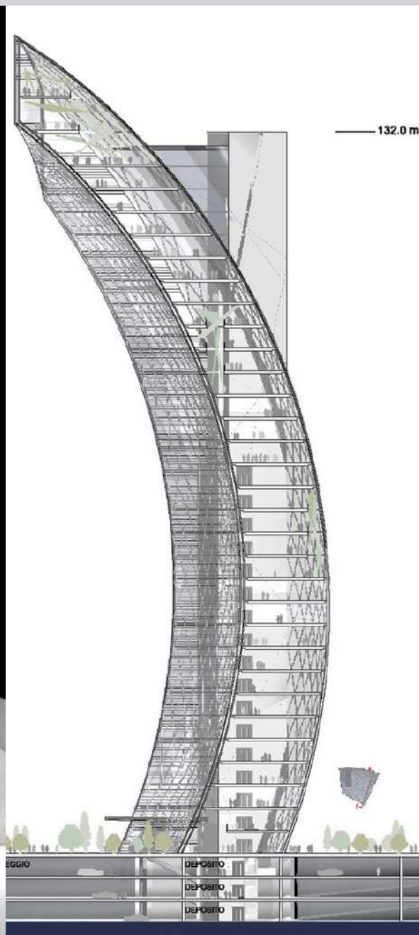
CITY LIFE LA TORRE - SEZIONE, VISTA DEL MODELLO DEFINITIVO
