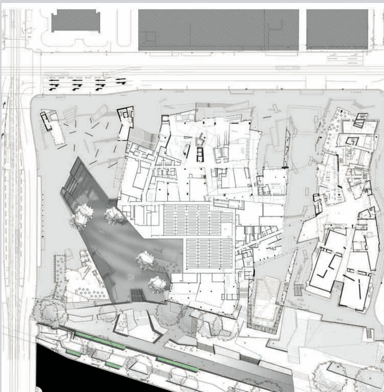
FD SQUARE- PLANIMETRIA A LIVELLO DI FLINDER STREET CON IL LABIRINTO PER LA PRODUZIONE DI ARIA FRESCA
