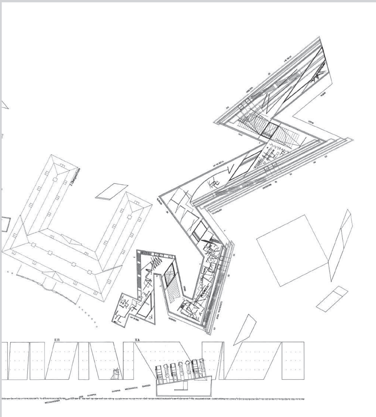
BERLIN MUSEUM -PLANIMETRIA PIANO SECONDO E SEZIONI PROGETTO DI CONCORSO
