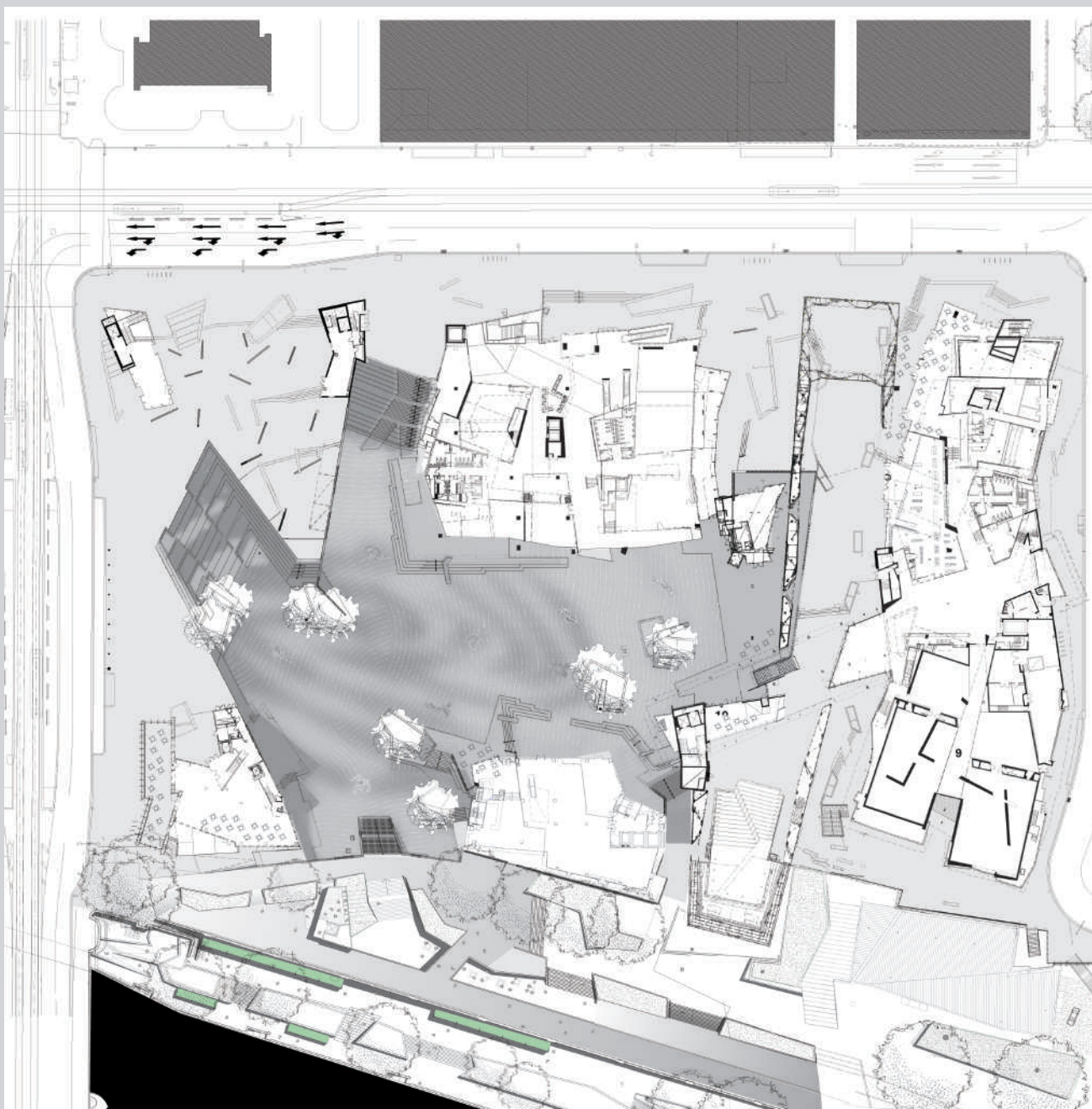
FD SQUARE - PLANIMETRIA A LIVELLO DELLA PIAZZA
